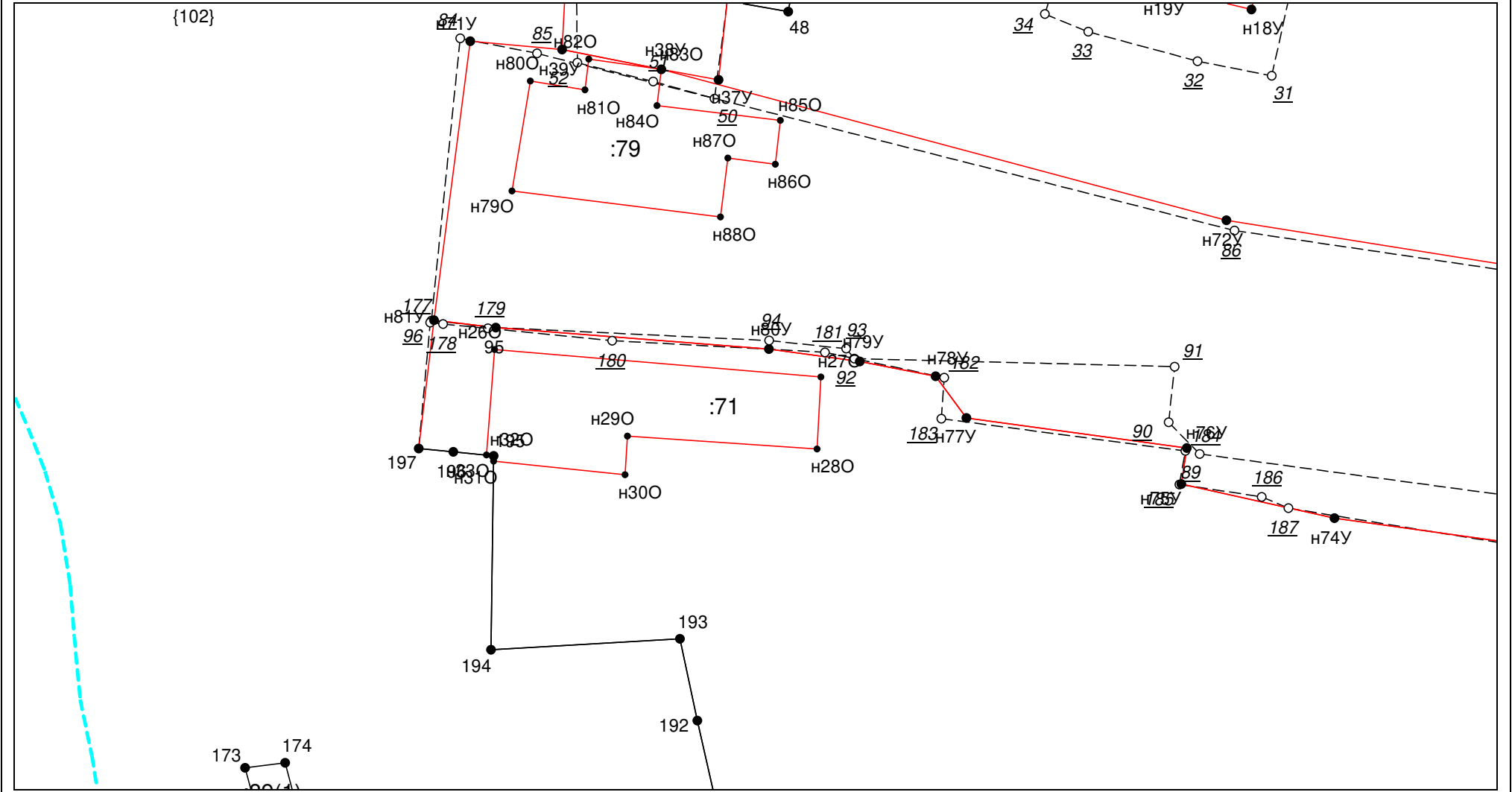
Выносной лист №12
